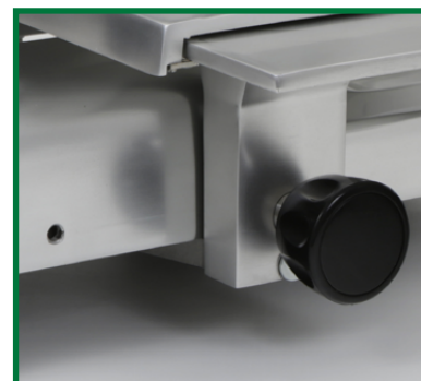
BLC - sistema blocco carro di scorrimento che consente di smontare il piatto e il suo supporto per avere così un comodo accesso nella parte sottostante per una più facile pulizia.
