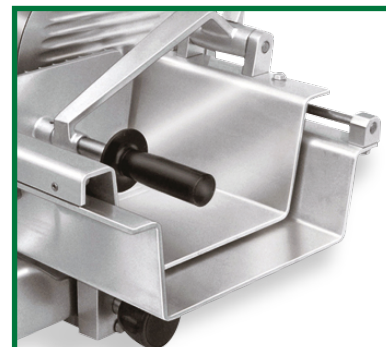
Piatto carni indicato per tagliare appositamente qualsiasi tipo di carne, di varie dimensioni, dalla forma a U per contenere anche le carni più morbide.
