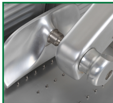
Ciabatta fissa in alluminio con puntine in acciaio inox ed ergonomico braccio pressamerce a cigno con puntine in acciaio inox.
